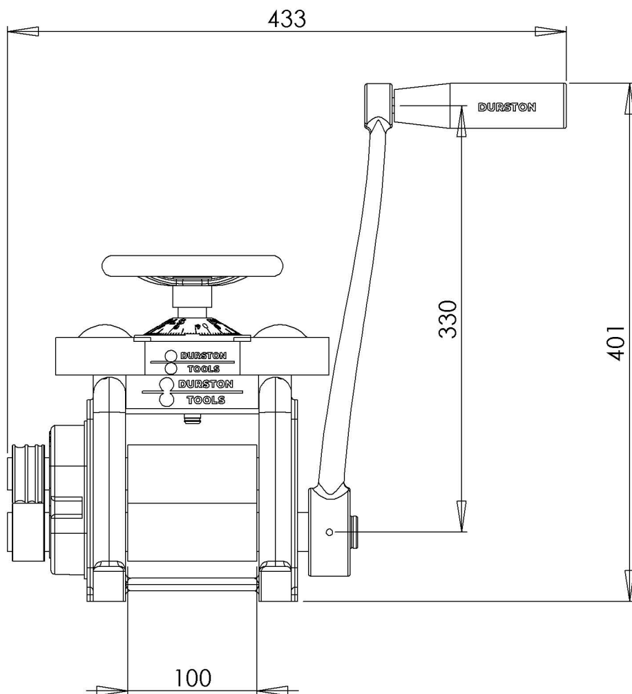
Mini C100E Rolling Mill SKU: 1003 Dimensions is MM
