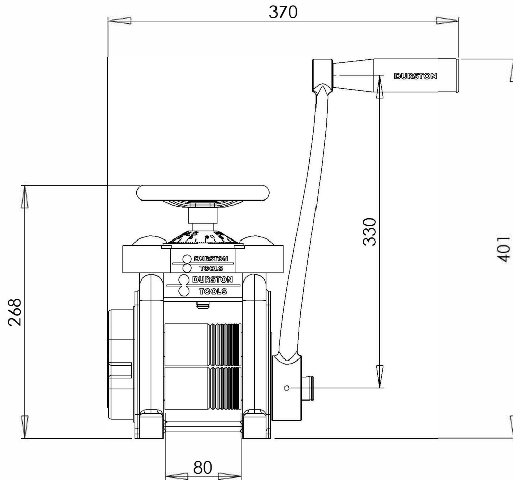
Mini C80 Rolling Mill SKU: 1000 Dimensions in MM
